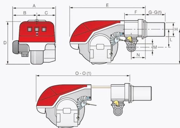
GRS 70 - 100 - 130 - 190 - 250
